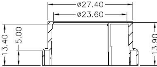
剖面圖 A-A
