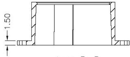
剖面圖 B-B
